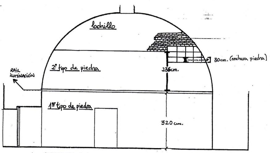
SECCION 1-1.
